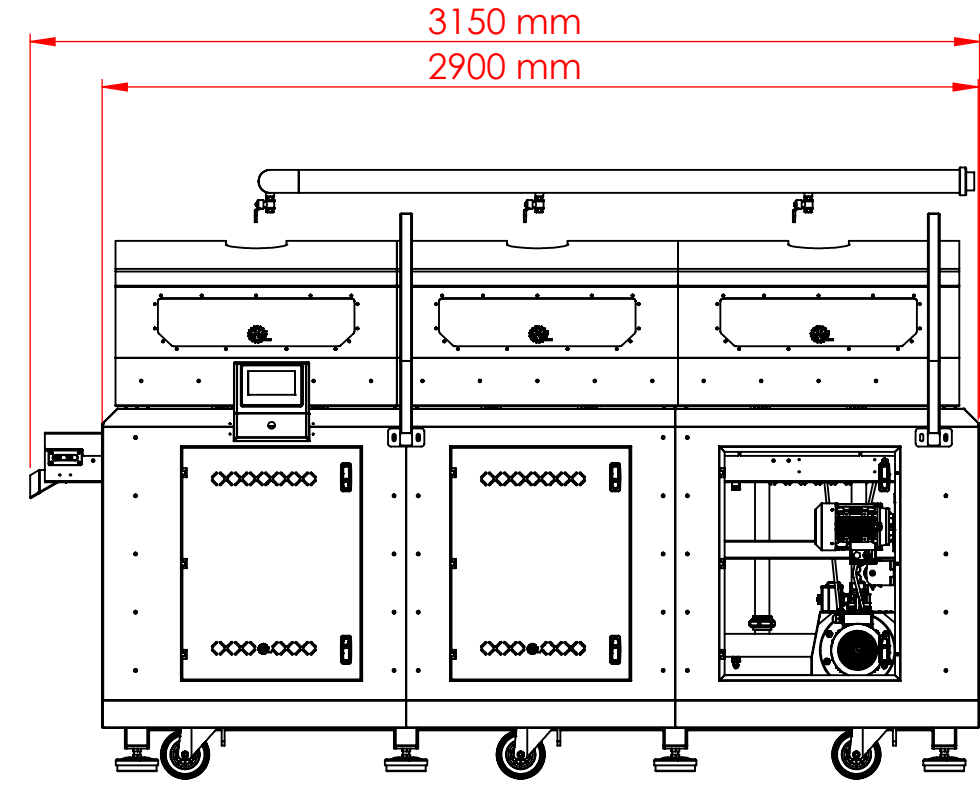
KESIT A-A
